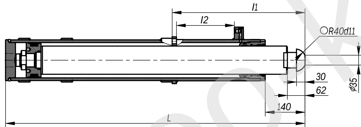
Рисунок 3 (1:2) Остальное - см. рисунок 1
